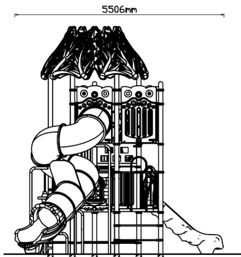
Vooraanzicht
