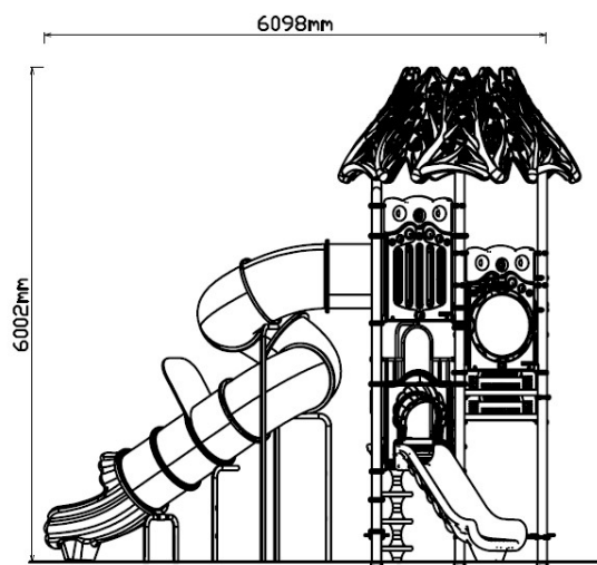
Zijaanzicht
