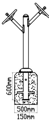
Zijaanzicht
