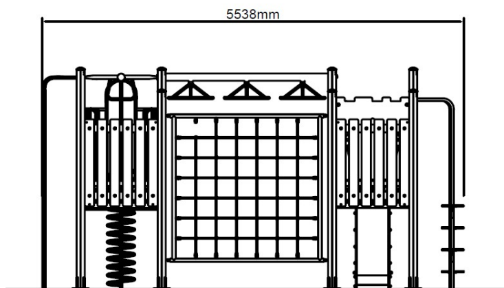
Vooraanzicht
