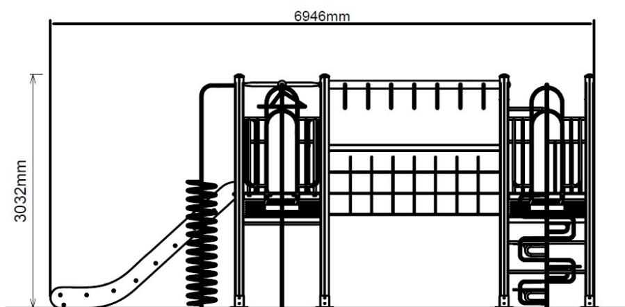
Zijaanzicht
