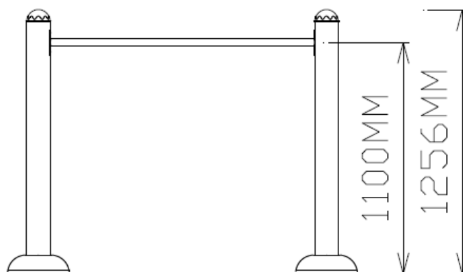
Vooraanzicht
