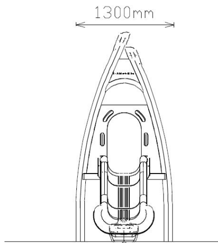
Vooraanzicht
