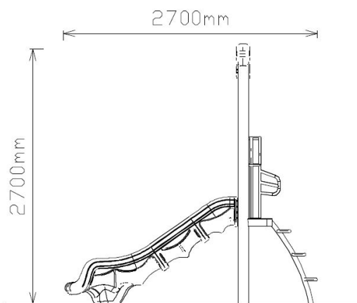
Zijaanzicht
