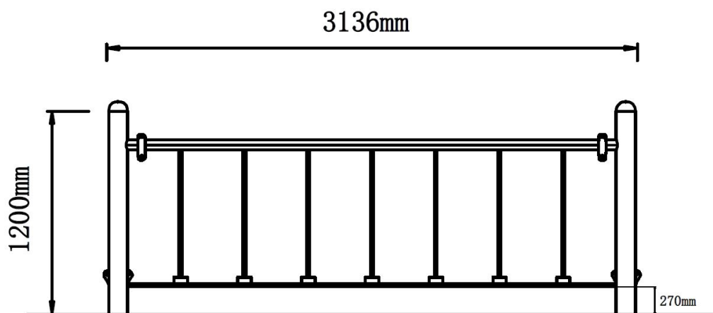
Vooraanzicht
