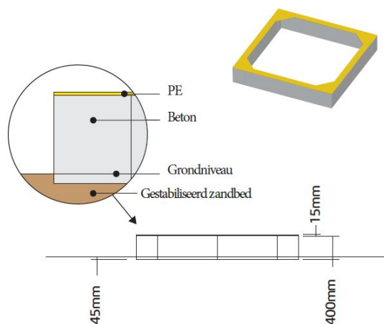
Vooraanzicht
