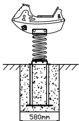
Zijaanzicht
