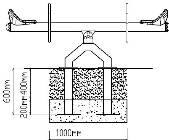
Zijaanzicht
