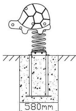
Zijaanzicht
