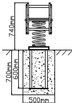
Vooraanzicht
