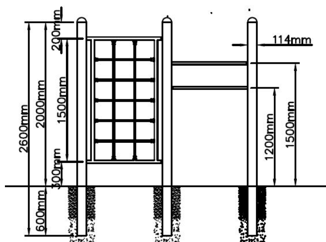
Zijaanzicht
