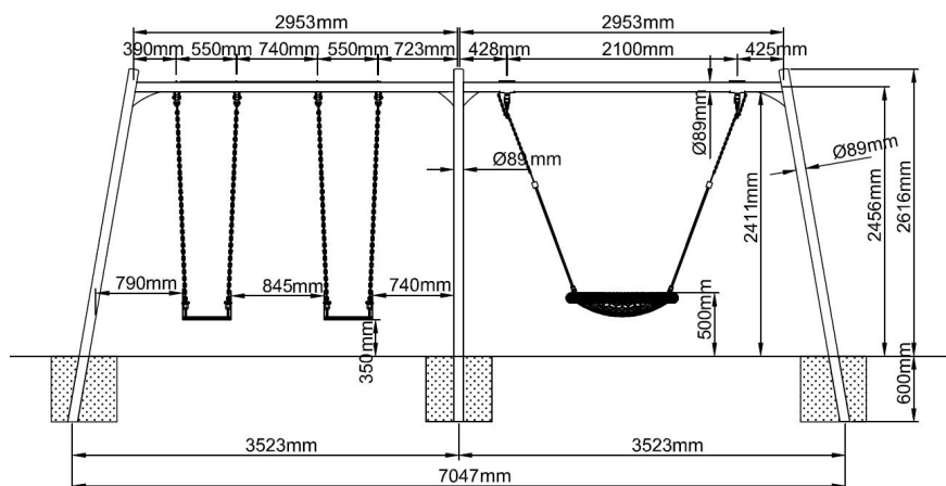
Vooraanzicht
