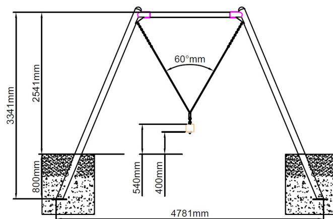
Vooraanzicht
