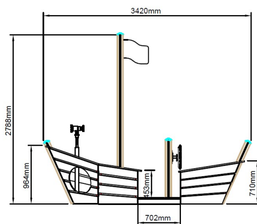
Zijaanzicht
