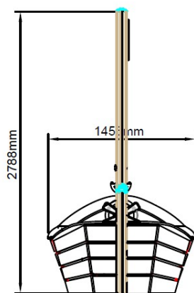
Vooraanzicht
