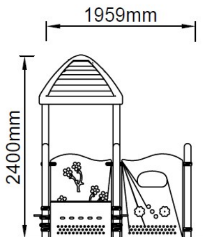
Vooraanzicht
