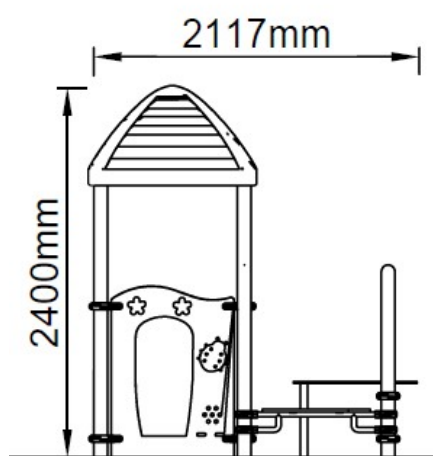
Zijaanzicht
