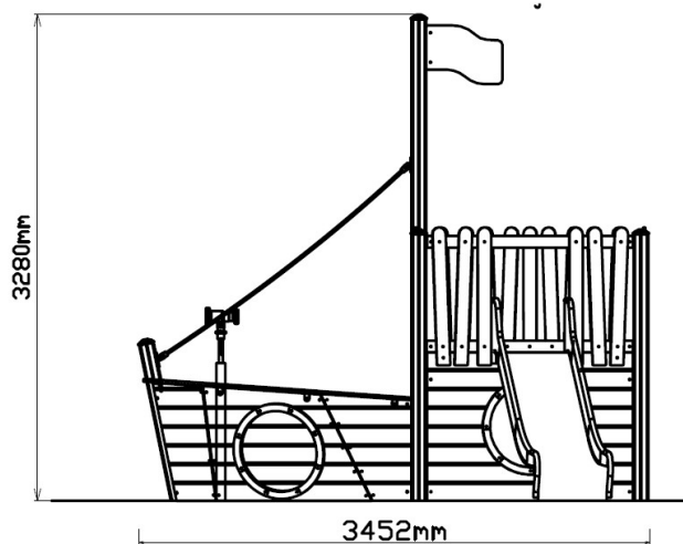
Vooraanzicht
