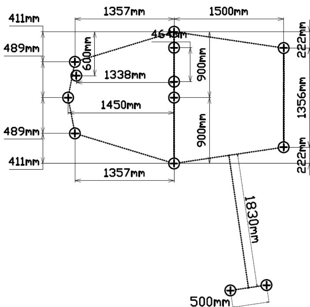
Plattegrond palenplan
