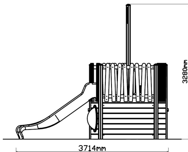
Zijaanzicht
