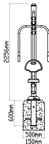
Vooraanzicht
