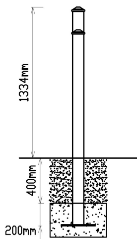
Zijaanzicht
