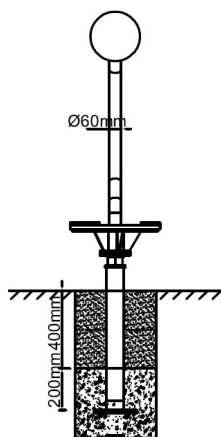
Zijaanzicht
